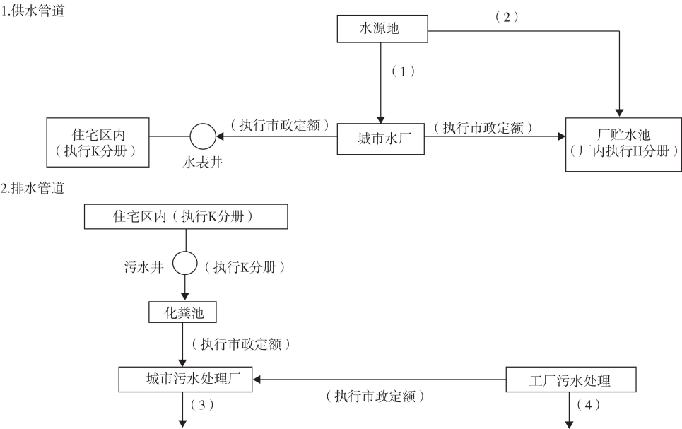
图 1-6 给排水管道定额执行分界线
